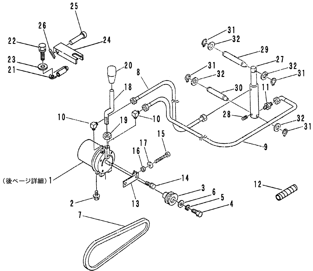
FIG 19 ユアツソウチ HYDRAULIC SYSTEM
