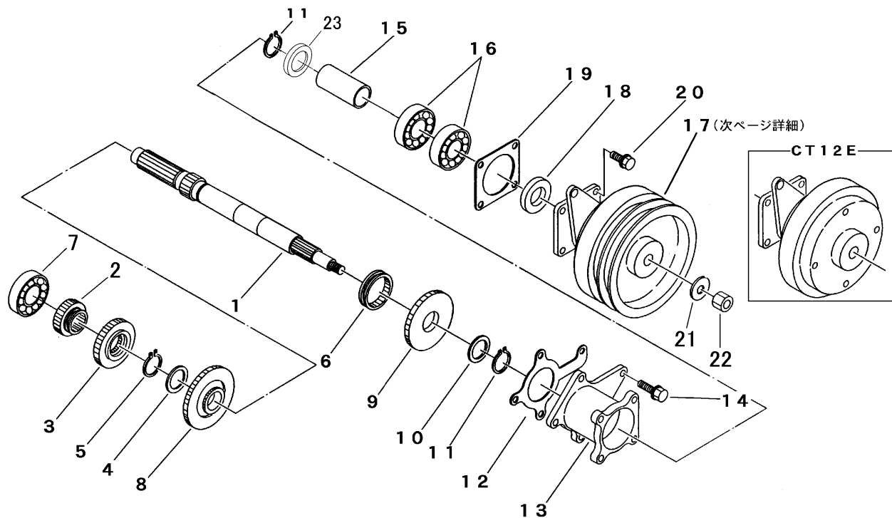
FIG 2 シャフト1 & クラッチ 1st SHAFT & CLUTCH
