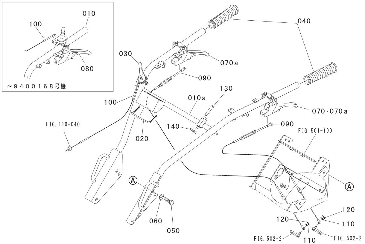
FIG. 505 ハンドル・サイドクラッチ・コントロールレバー
