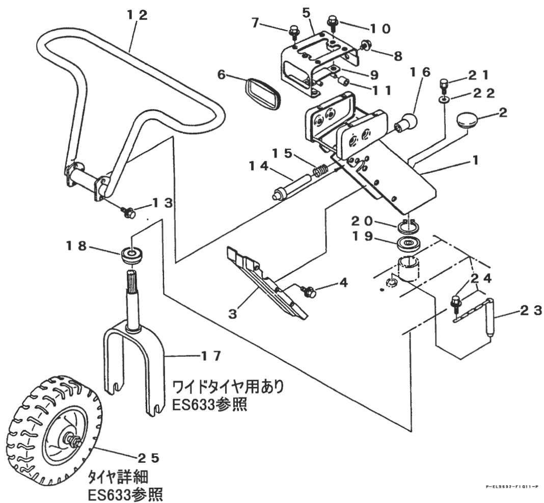
FIG 11 ハンドル HANDLE
