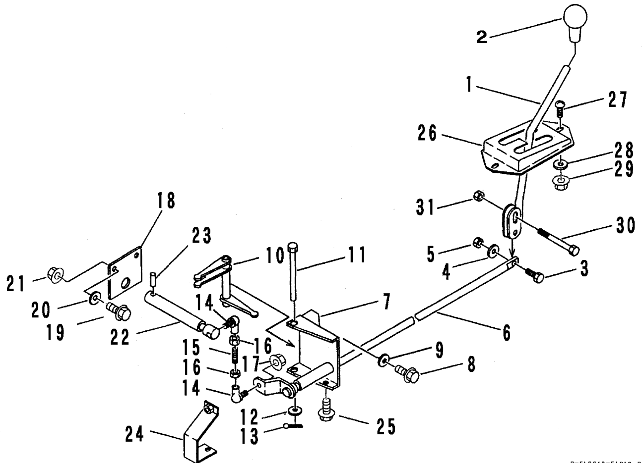
FIG 9 チェンジレバー LEVER
