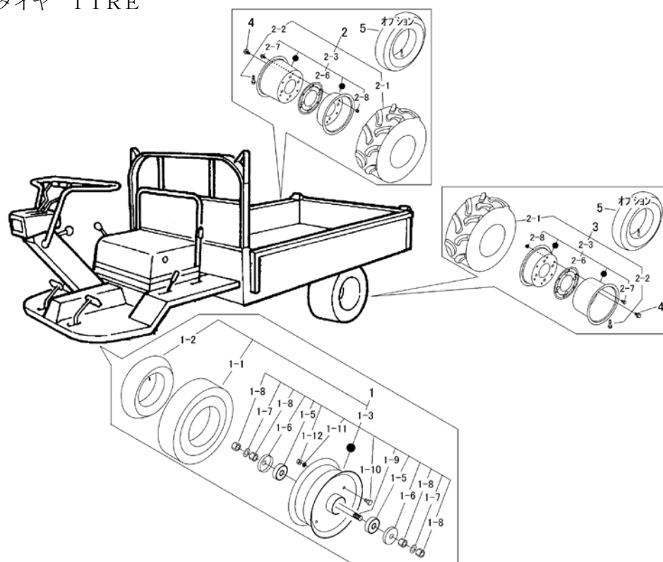
FIG 7 タイヤ TIRE
