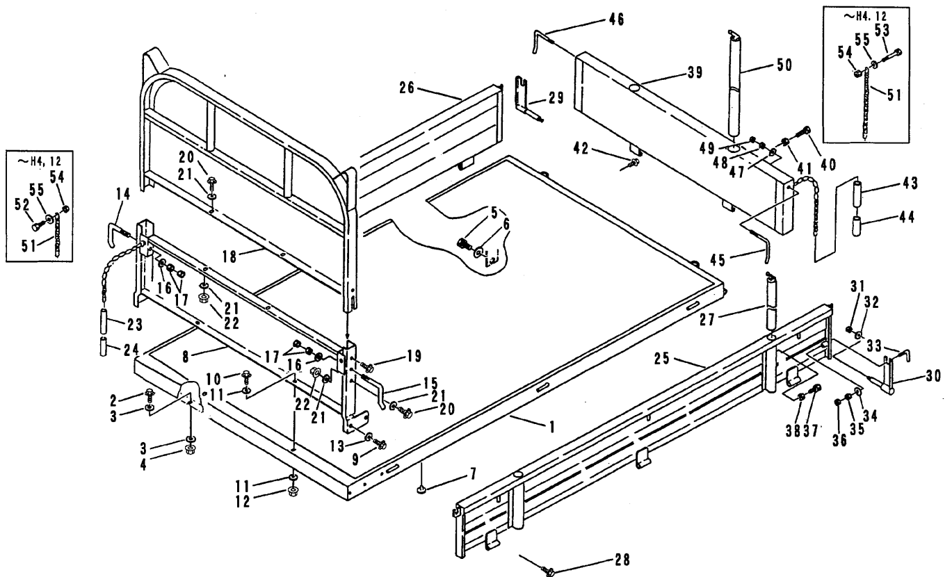
FIG 12 ニダイ&ドア WAGON&GATE (標準荷台)
