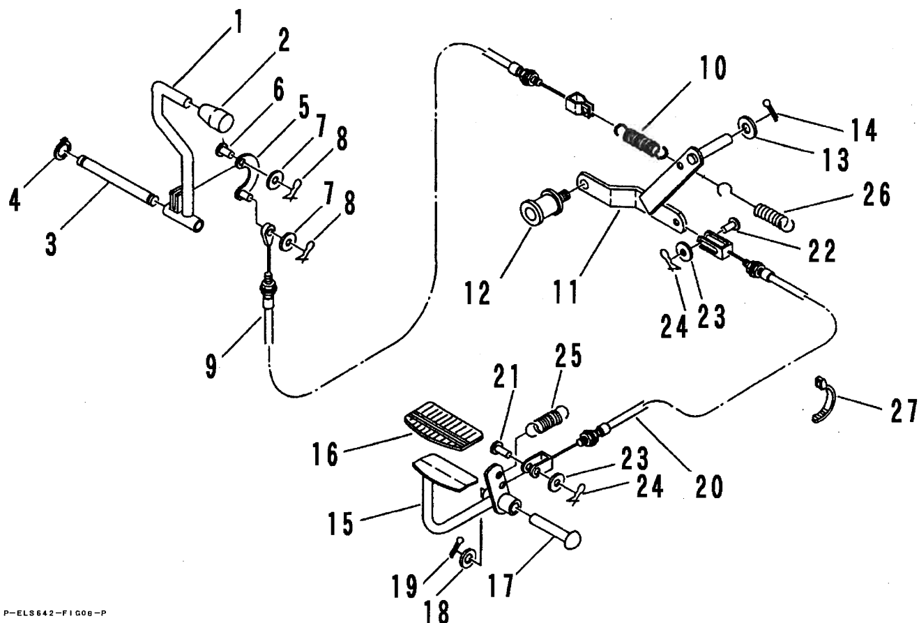
FIG 7 クラッチレバー LEVER
