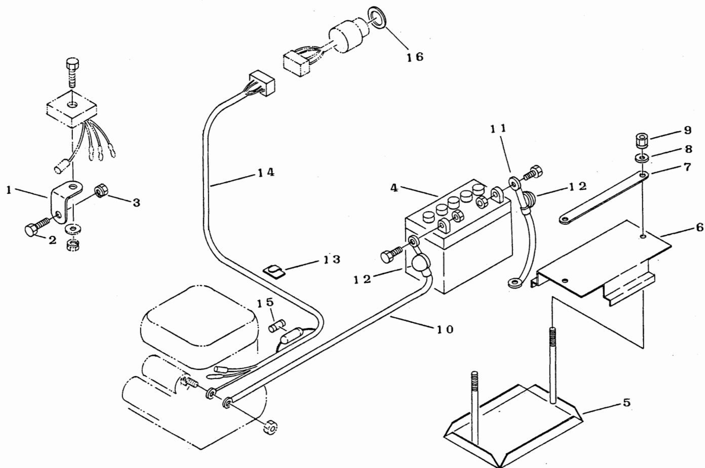
Fig 2 バッテリー 仕様 BATTERY
