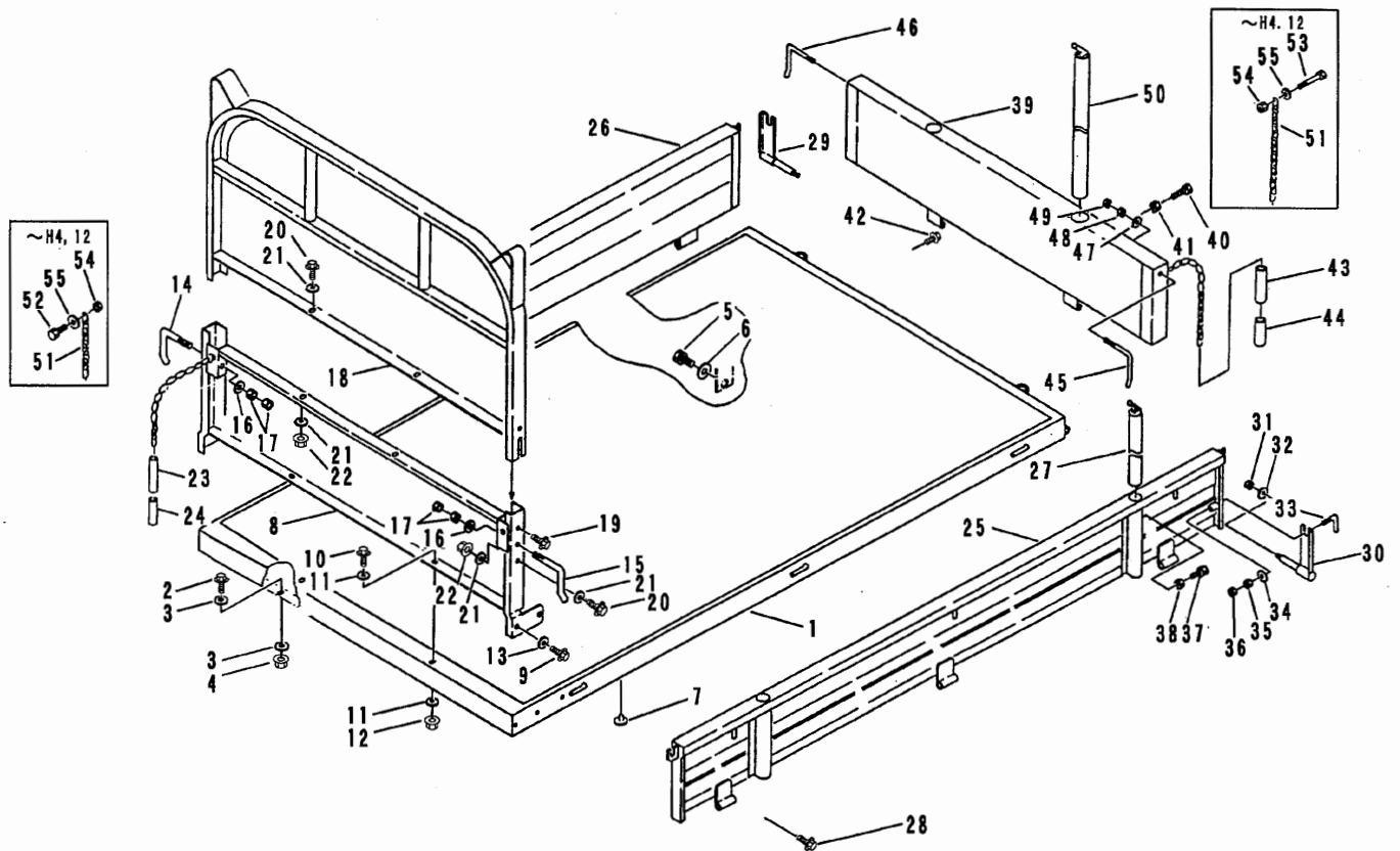
FIG 13 ニダイ&ドア WAGON&GATE (標準荷台)
