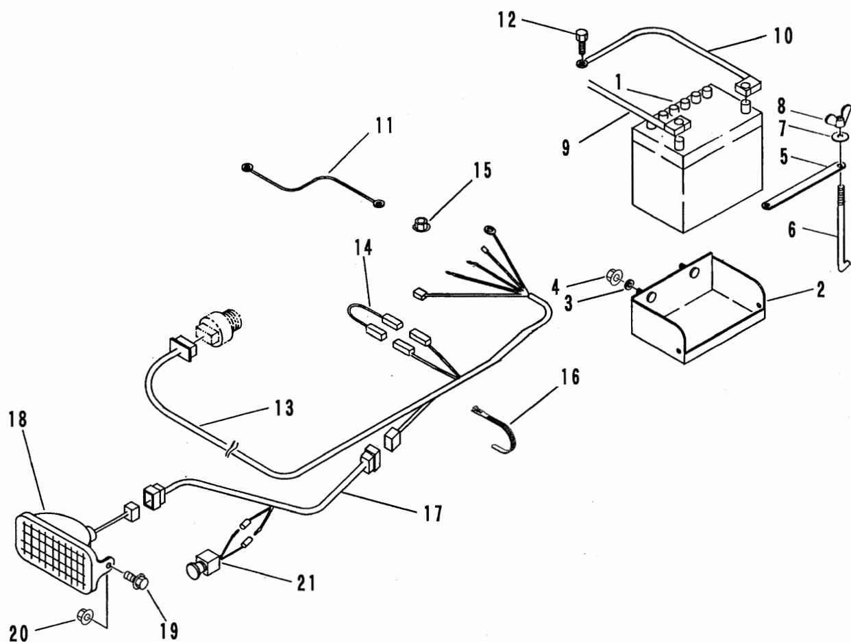
FIG 4 デンソー ELECTRIC クボタOC62
