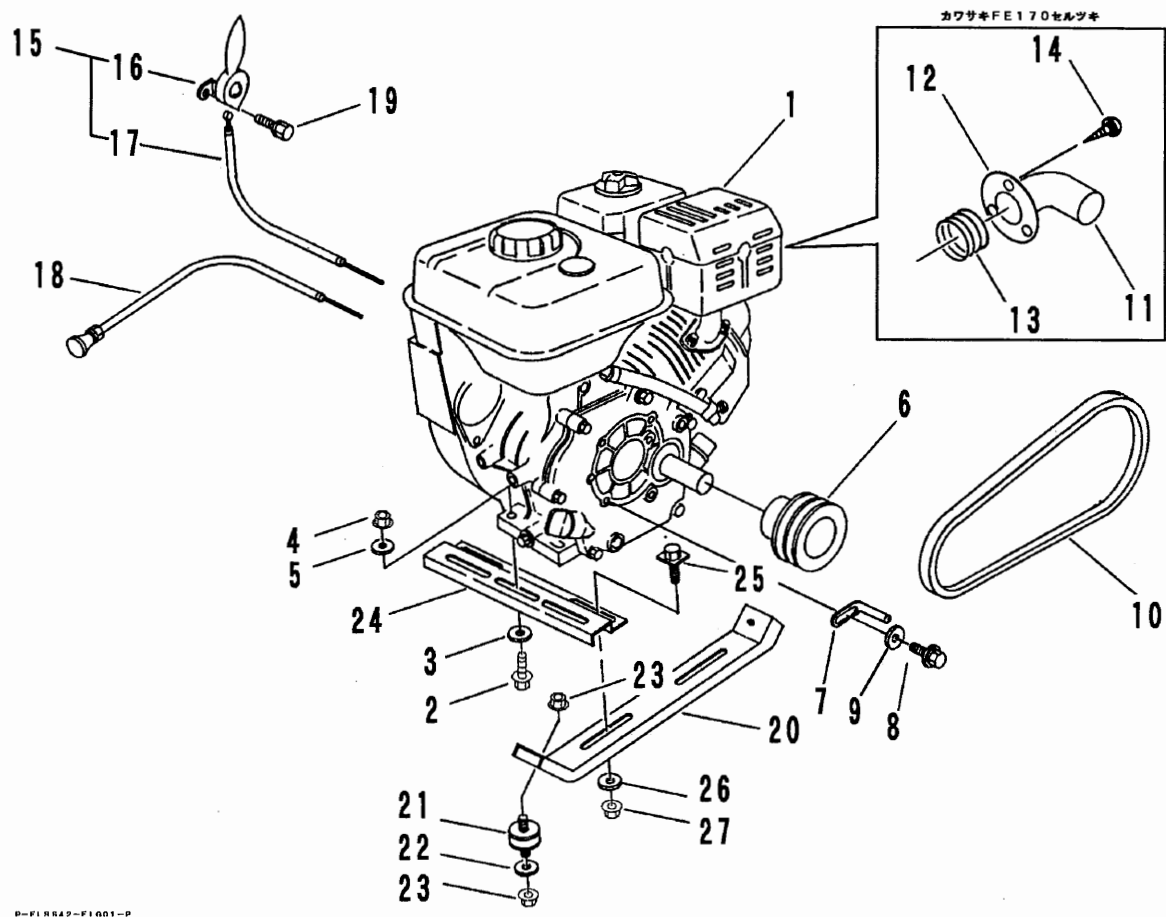
FIG 1 エンジン ENGINE ガソリン
