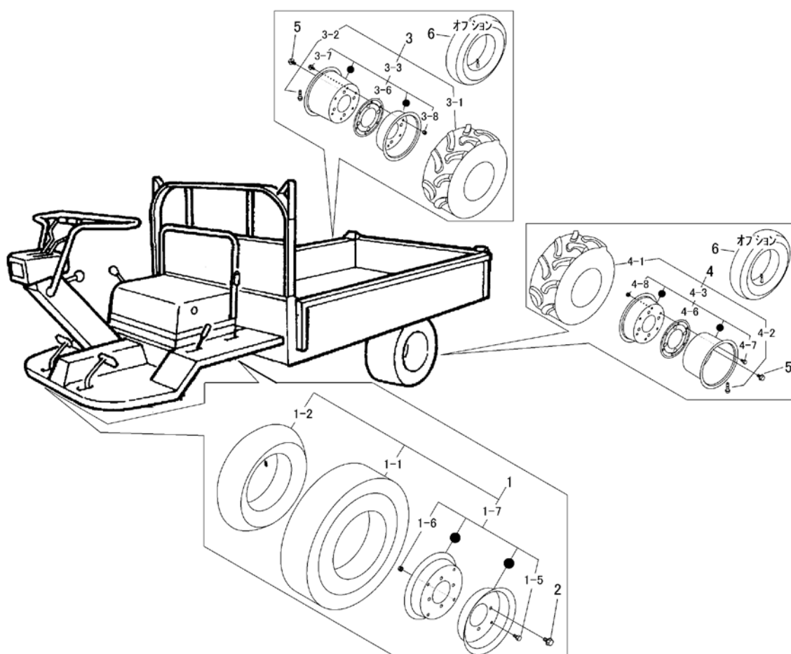
FIG 8 タイヤ TIRE
