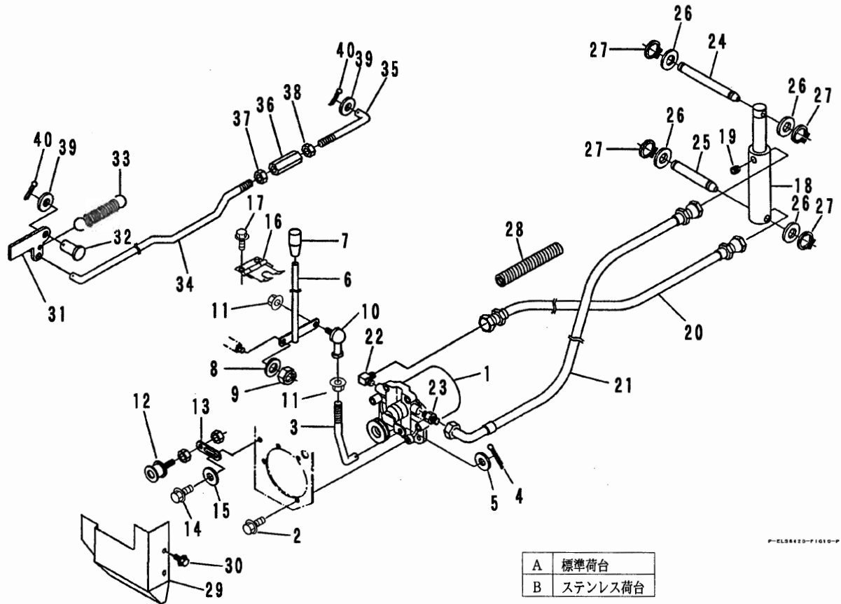
FIG 15 パッケージ HYD.PUMP
