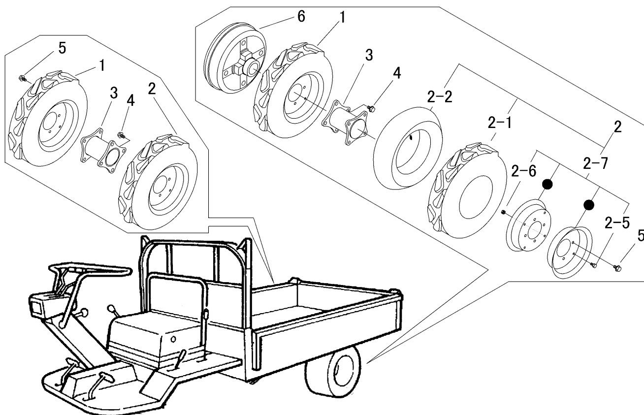
FIG 20 Wタイヤ TIRE (OPTION)
