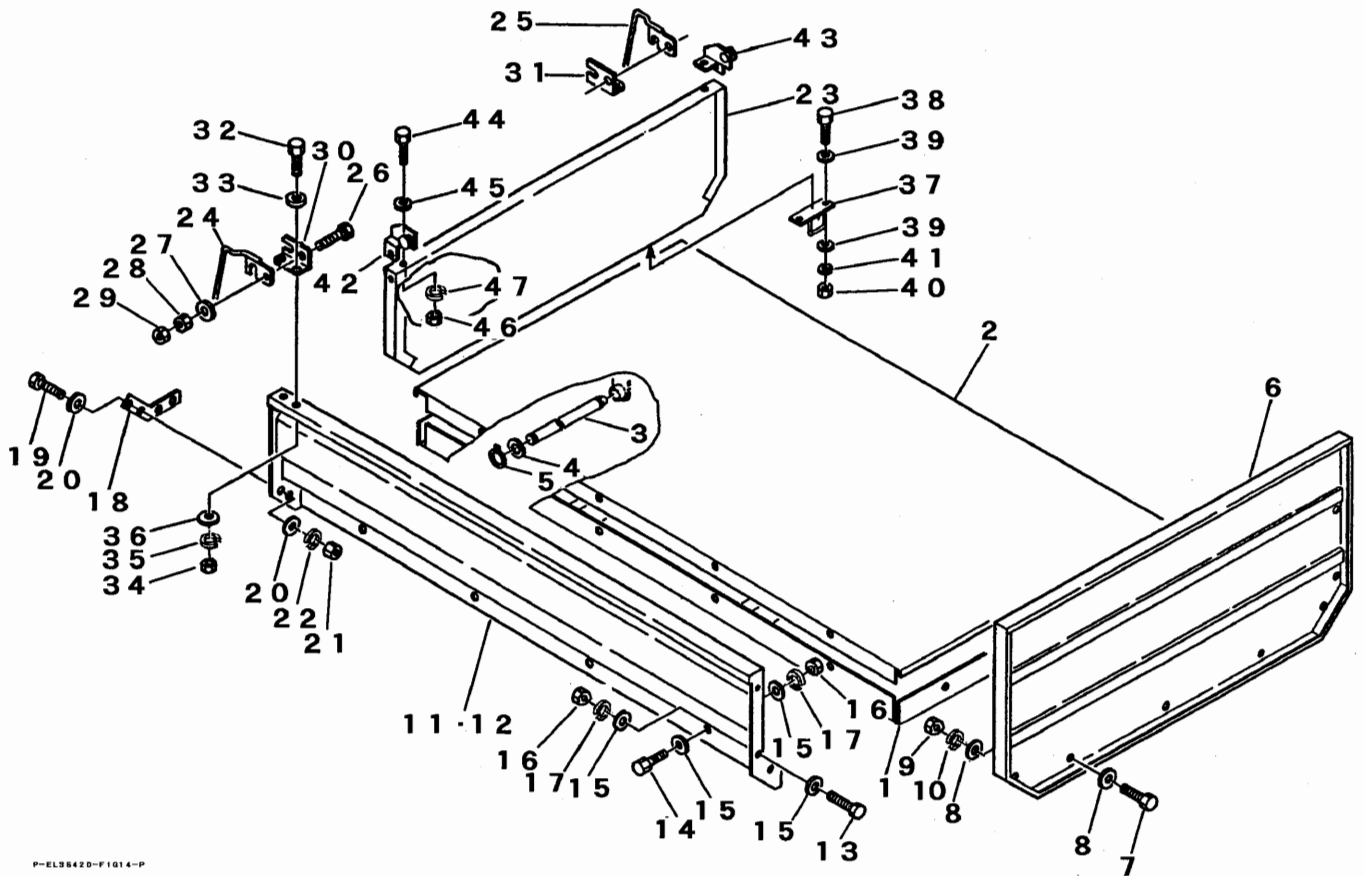
FIG 14 ステンレスニダイ WAGON
