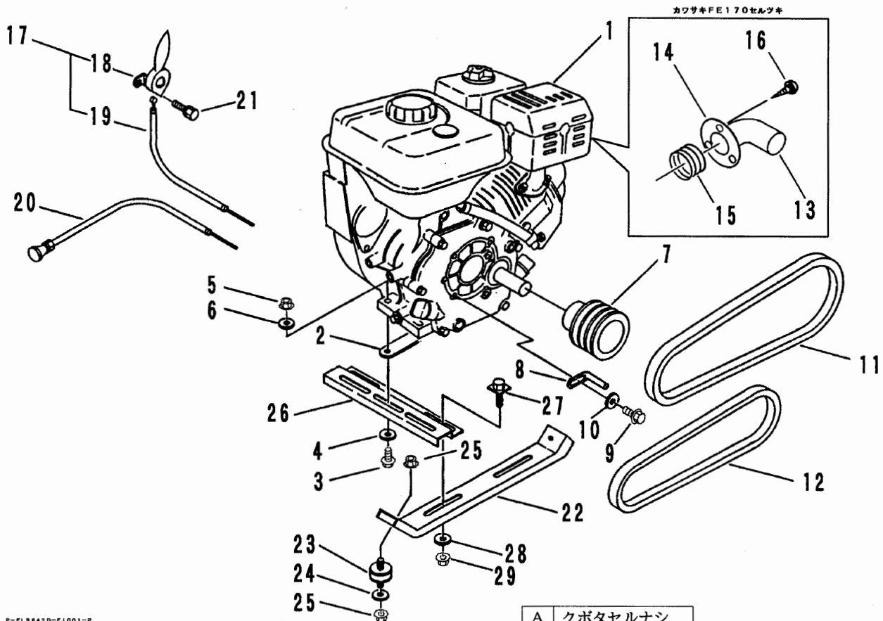
FIG 1 エンジン ENGINE ガソリン
