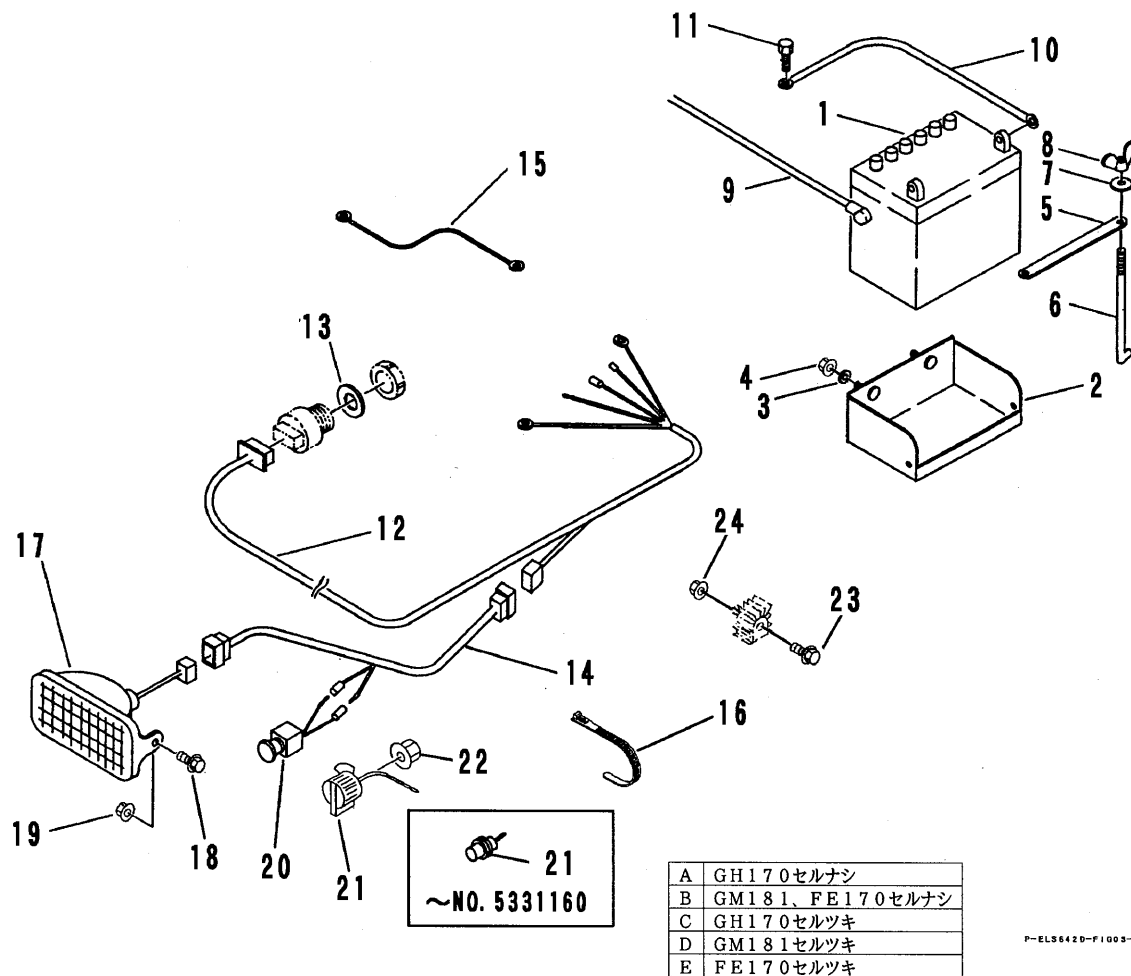
FIG 3 デンソウ ELECTRIC ガソリン
