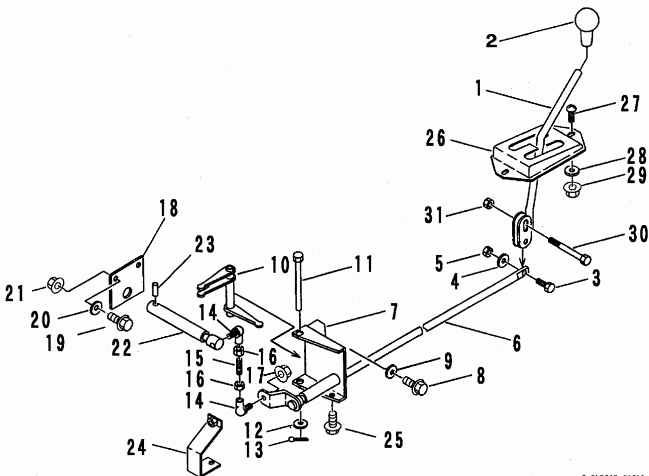
FIG 10 チェンジレバー LEVER
