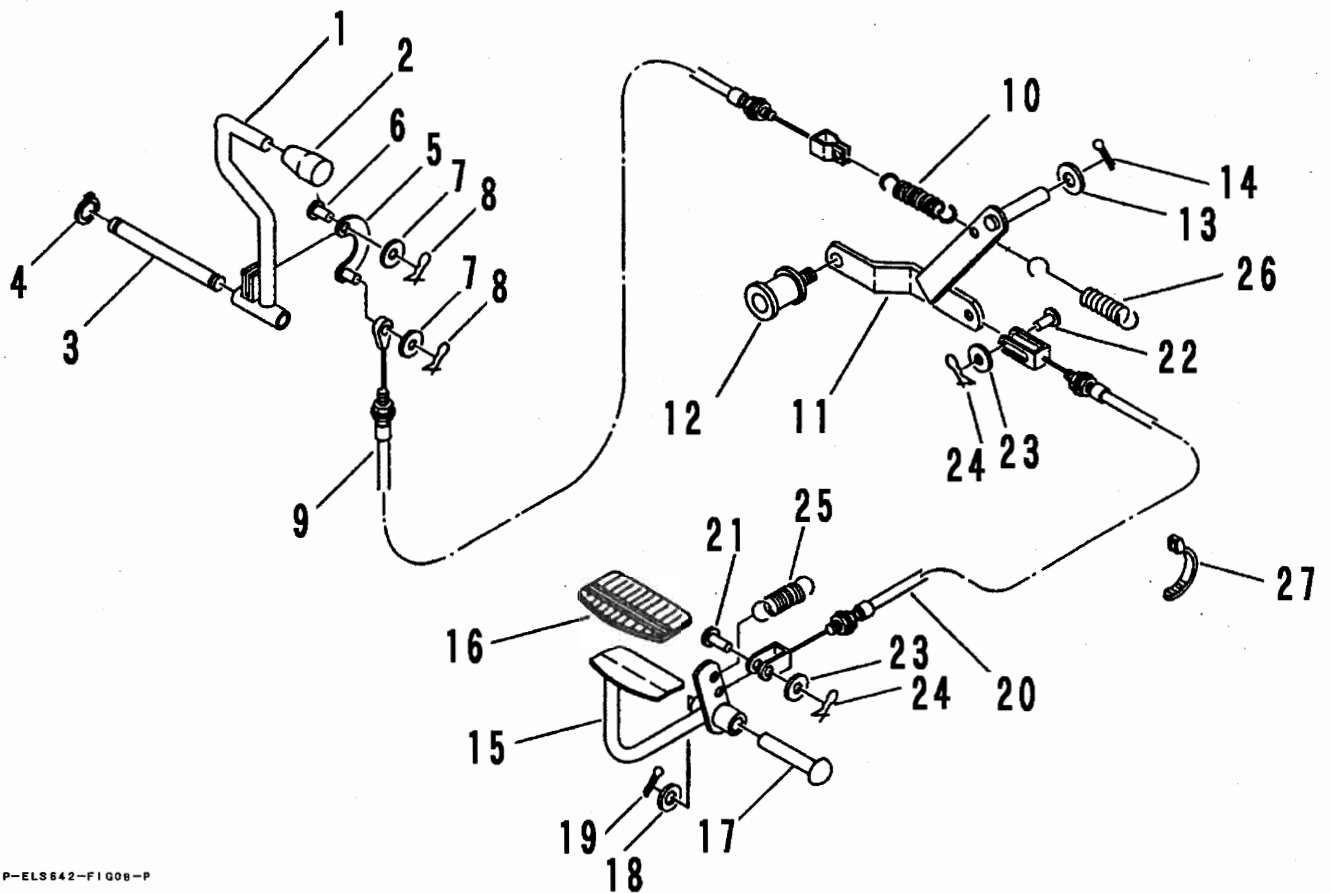
FIG 8 クラッチレバー LEVER
