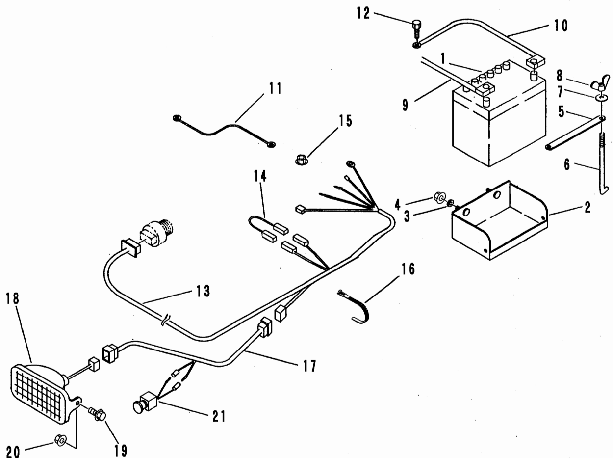
FIG 4 デンソウ ELECTRIC OC62
