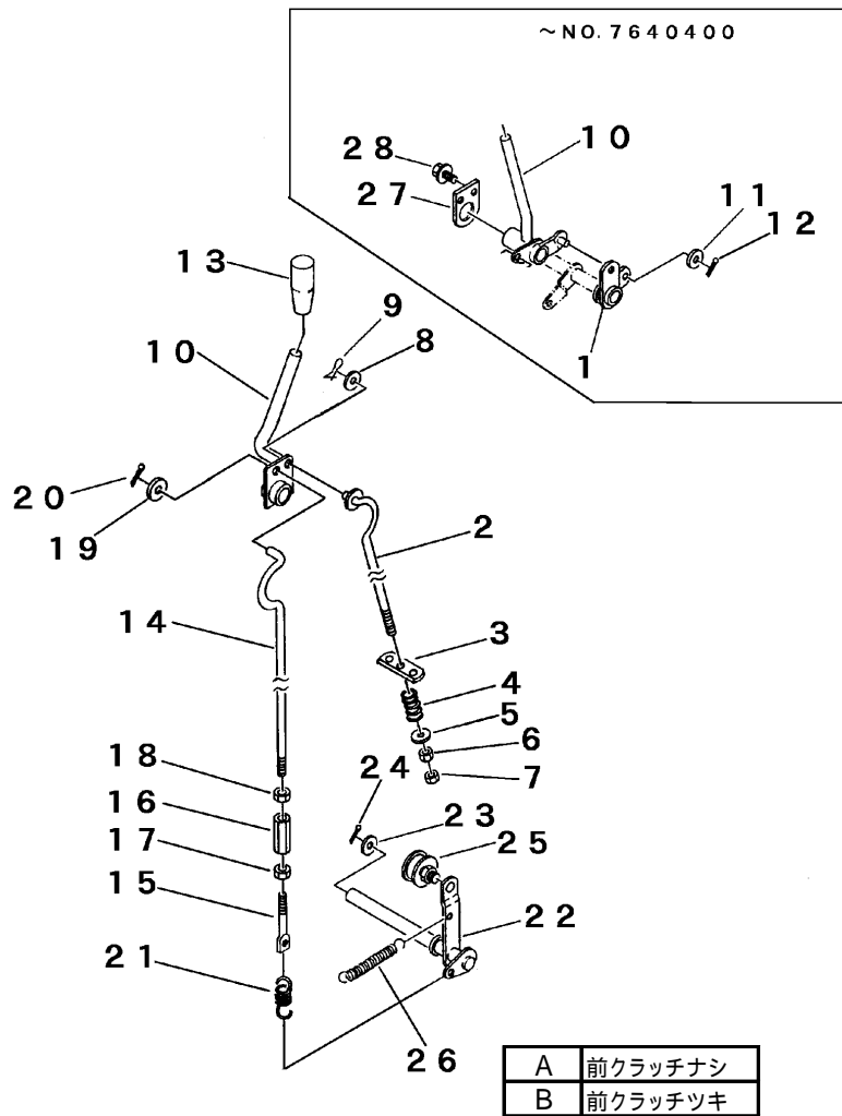
FIG 6 クラッチ & ブレーキレバー CLUTCH & BRAKE LEVER
