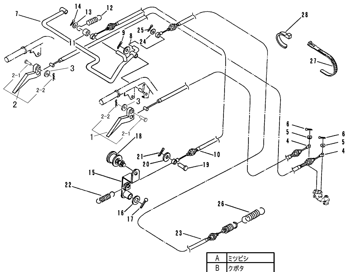
FIG 5 サイドクラッチ & クラッチ・ブレーキ SIDE CLUTCH & CLUTCH·BRAKE
