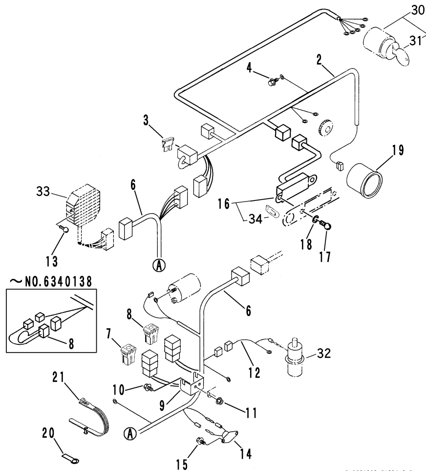
FIG 5 デンソウ (ソノ2) ELECTRIC EQUIPMENT (PART - 2)
