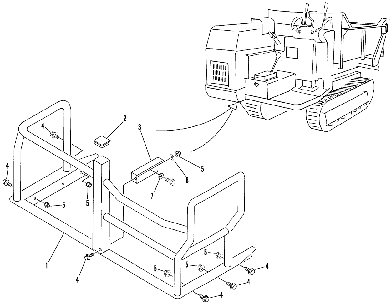
FIG 29 ウンテンセキガード (オプション) CAB GUARD (OPTION)
