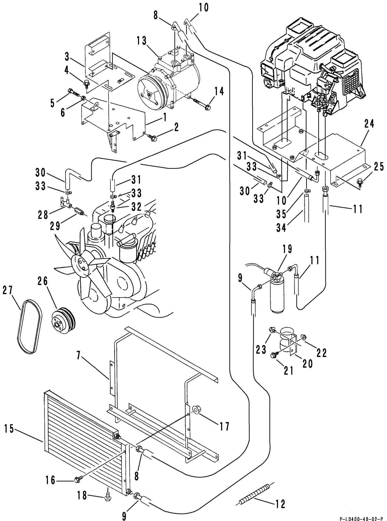
エアコン (ソノ 1) オプション FIG 40 AIR-CON (PART-1) OPTION
